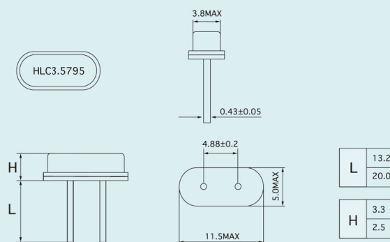
49U/S DIMENSIONS(MM)
